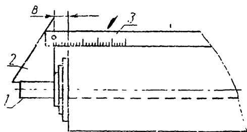
1—шпуля, 2—угольник, 3—линейка
