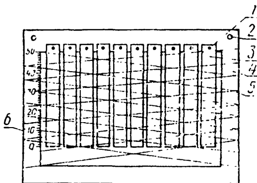
1—штыки для крепления образцов; 2—отверстия для крепления рамки в термостате или туннельной печи, 3—испытываемые образцы; 4—рамка; 5—нити; 6—шкала
